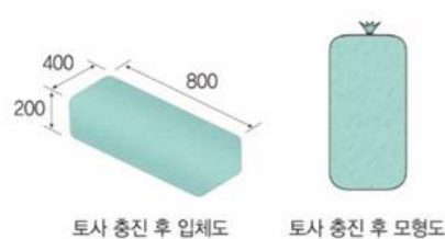
토사 충전 후
