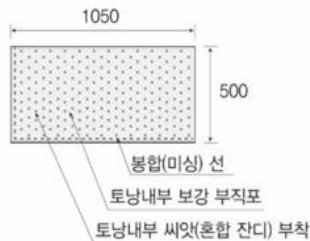
흙 채우기 전 식생토낭 규격(기본형)
