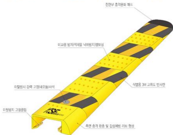
지게차 포크안전 커버 주요 구성도
